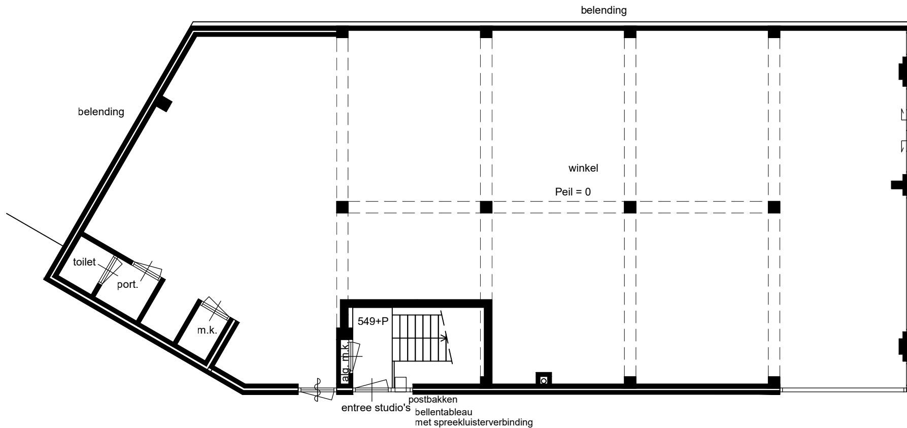
begane grond
